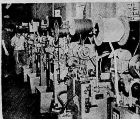
Aquí observamos algunas de las máquinas que fabrican los dientes y los adhieren a la cinta.
